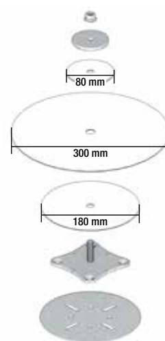
MAPEPLAN® ANCHORING INOX PLUS
